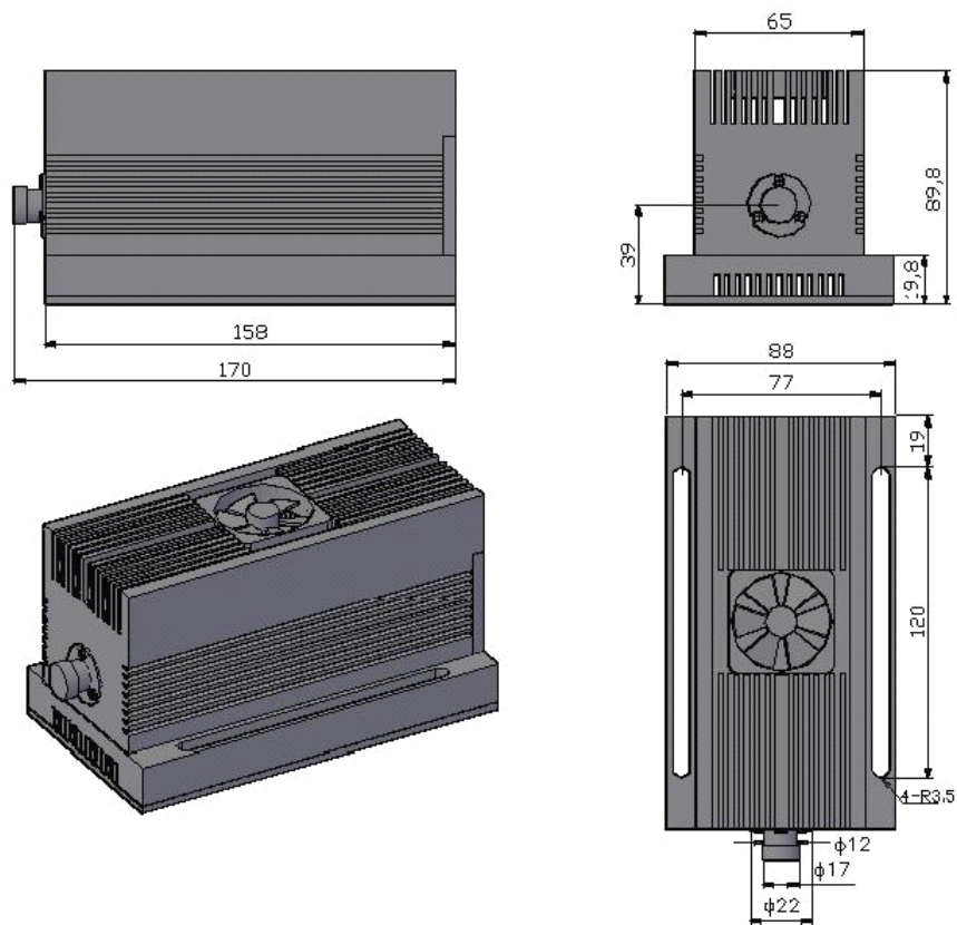
2.5-4W 532nm 激光头尺寸
