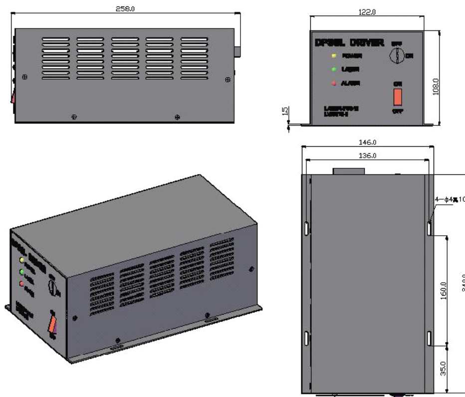
2.5-4W 532nm 激光电源尺寸 (10A)
